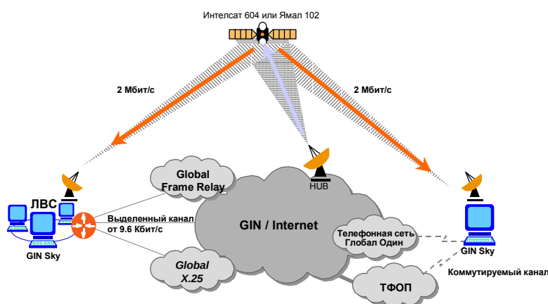
Схема подключения к сети GIN
